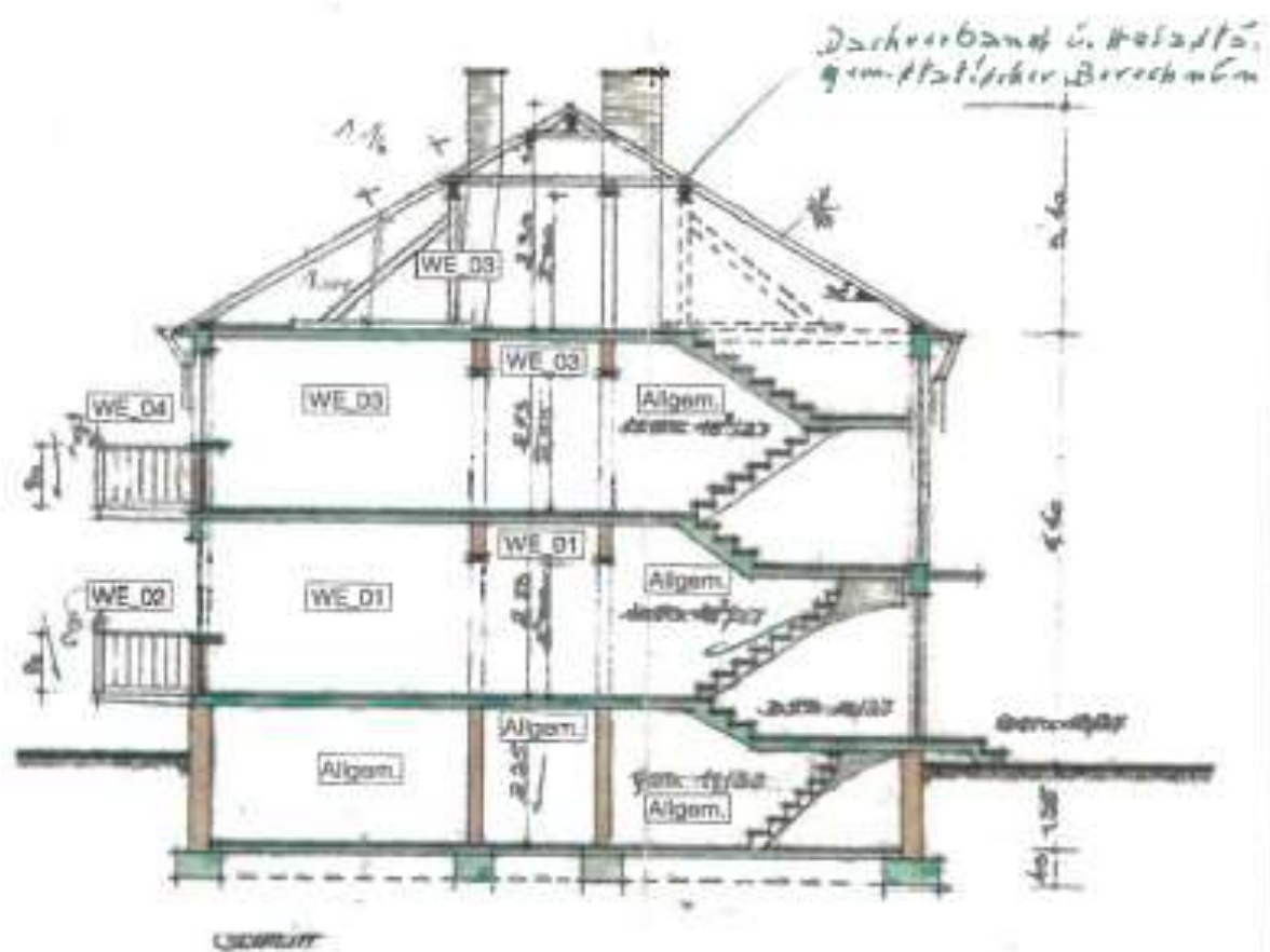
Schnitt
