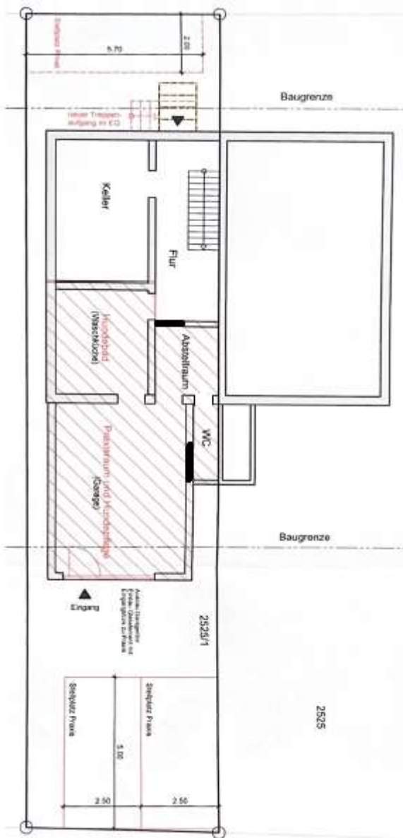
Untergeschoss
