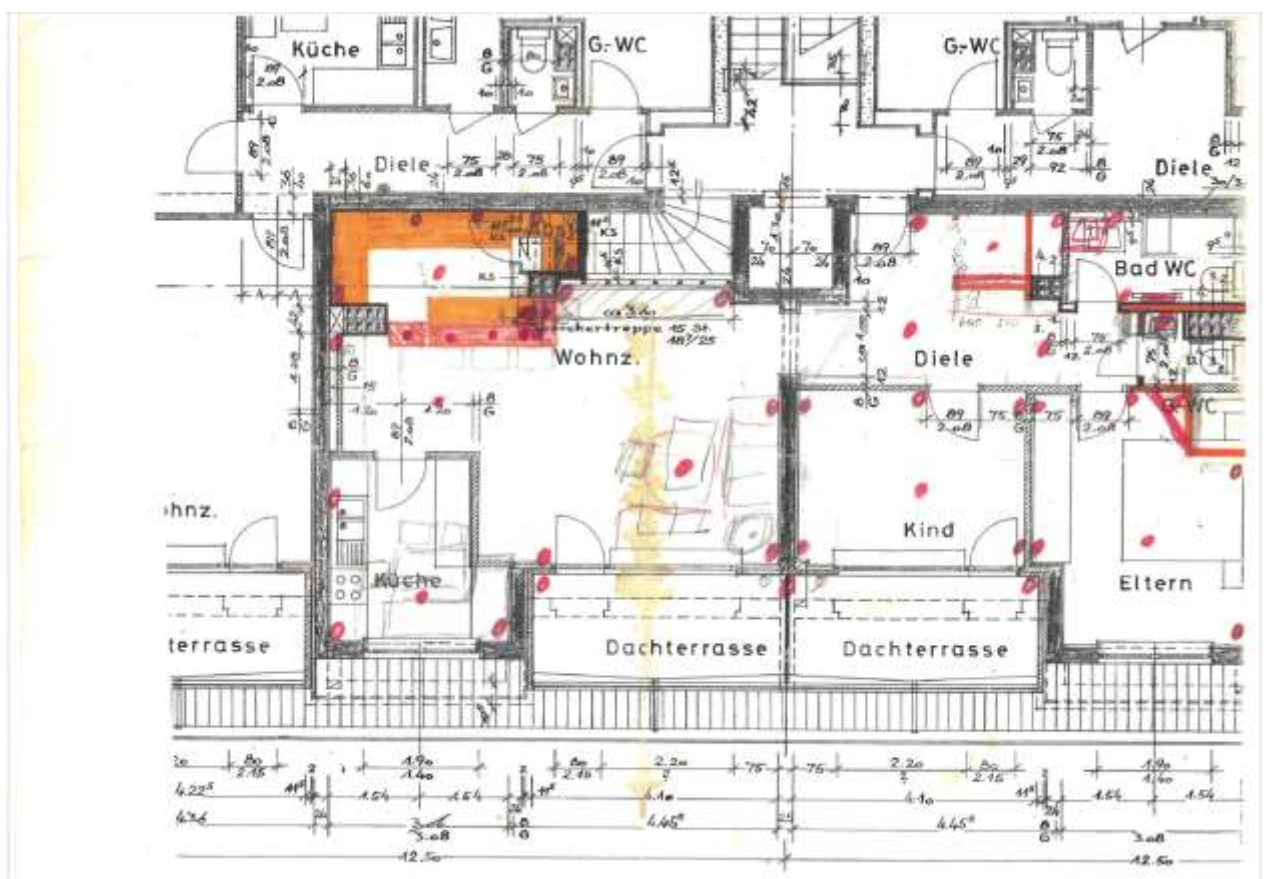
Grundriss
