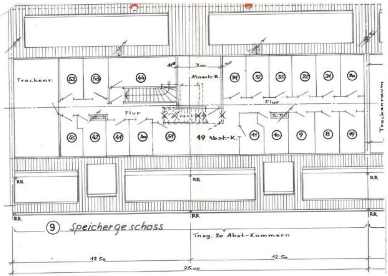
Grundriss
