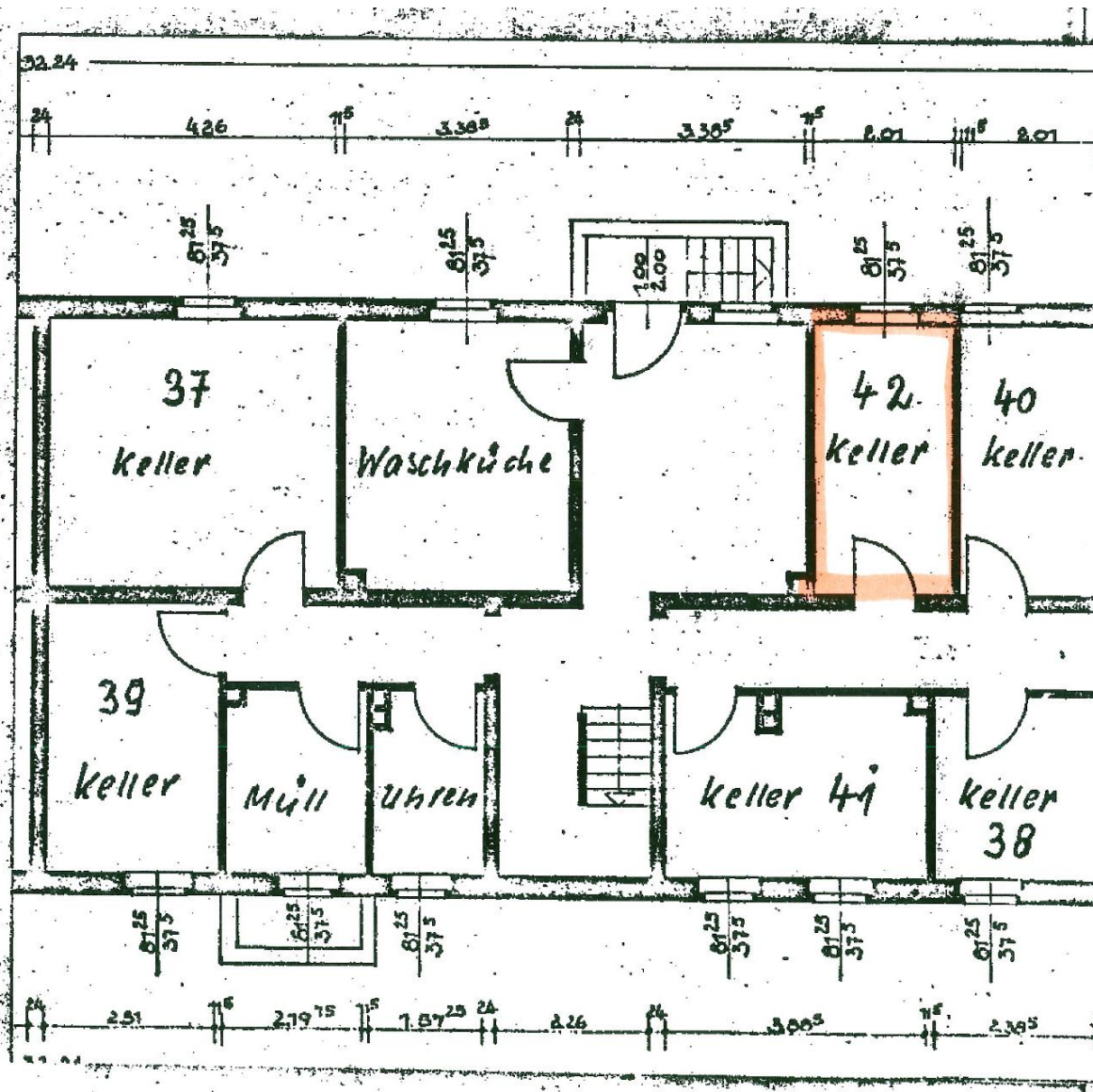
Grundriss Keller
