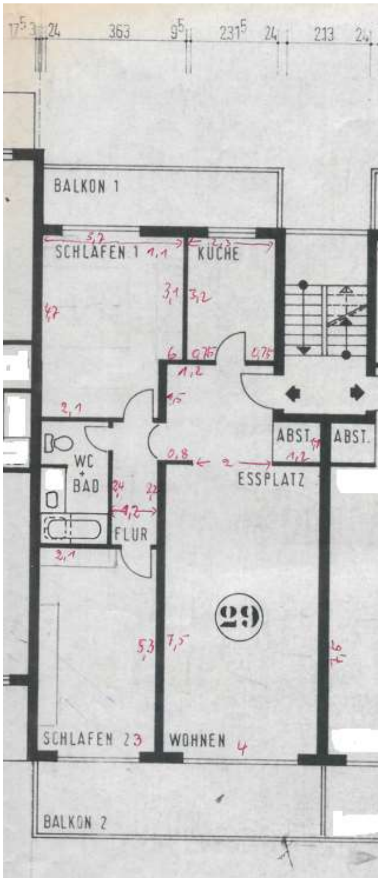
Grundriss Wohnung
