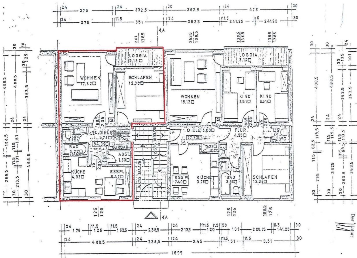
Grundriss Wohnung
