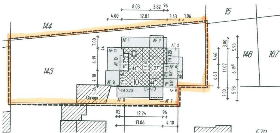
Lageplan
