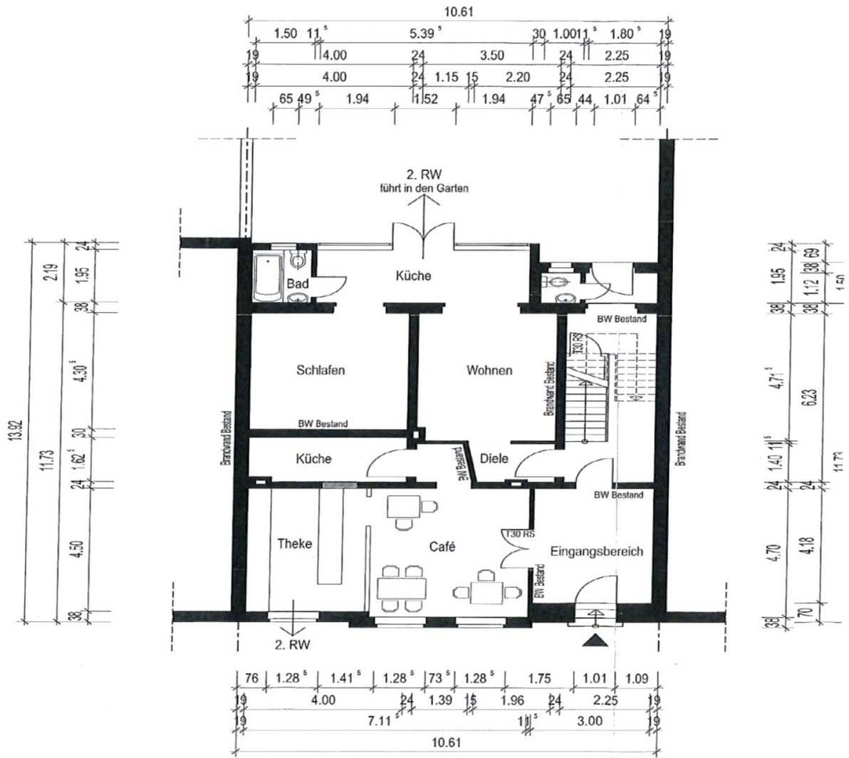
Grundriss Erdgeschoss
