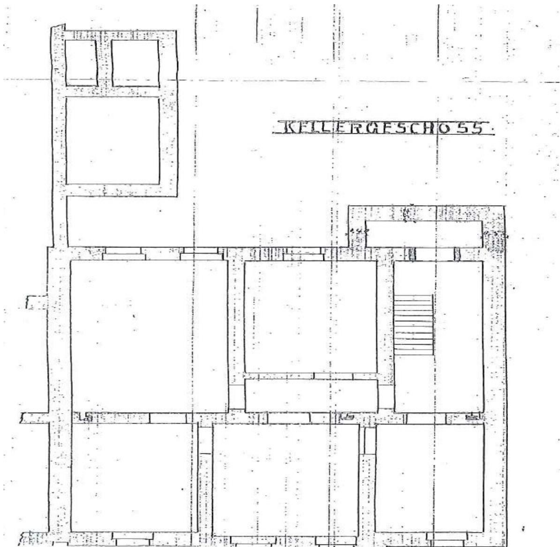
Kellergeschoss
