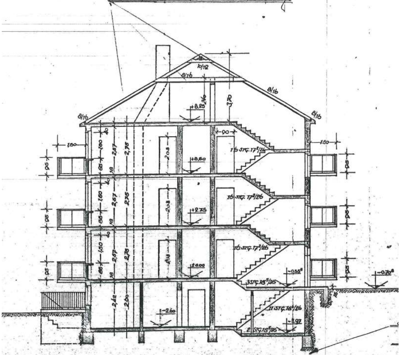
QUERSCHNITT DRITTEGESCHOSSIGER TEIL
