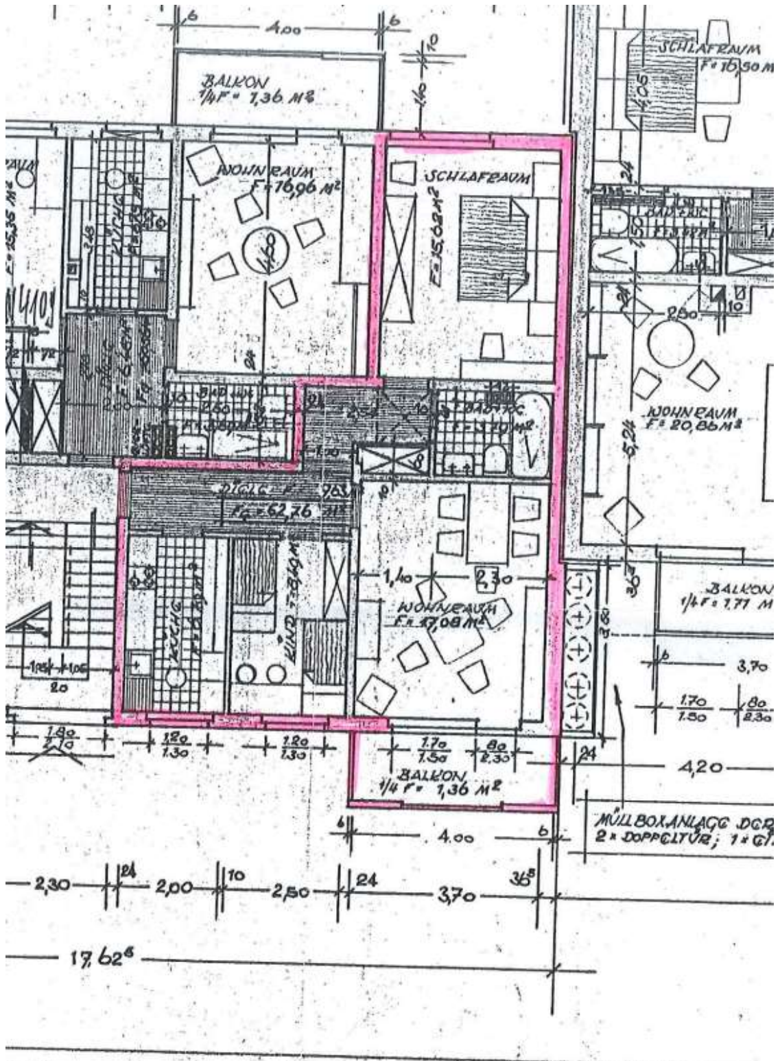
Grundriss Wohnung
