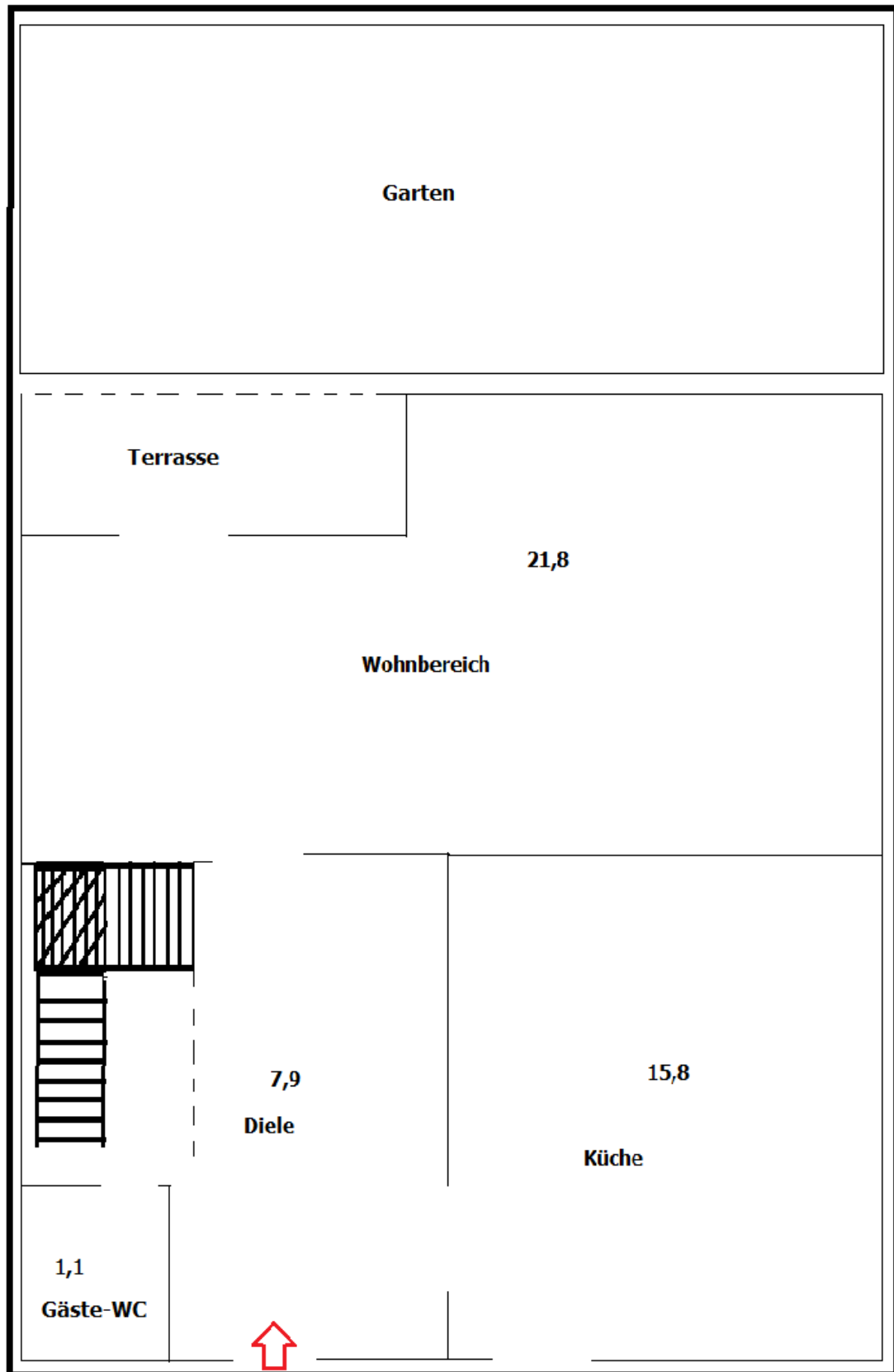
Grundriss Erdgeschoss
